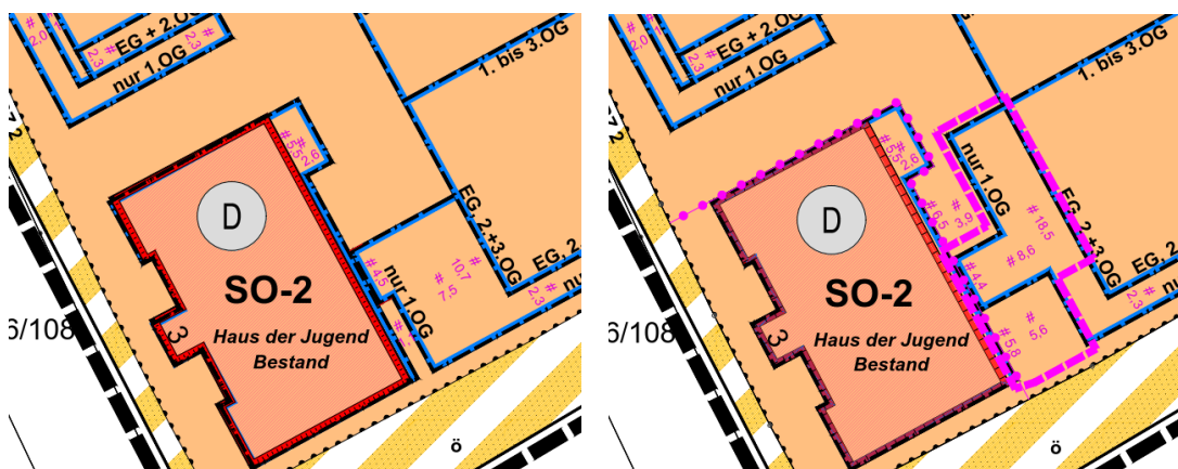
Abb. 7: Anpassung der Baugrenzen im ersten Obergeschoss – Vergleich vorher / nachher
