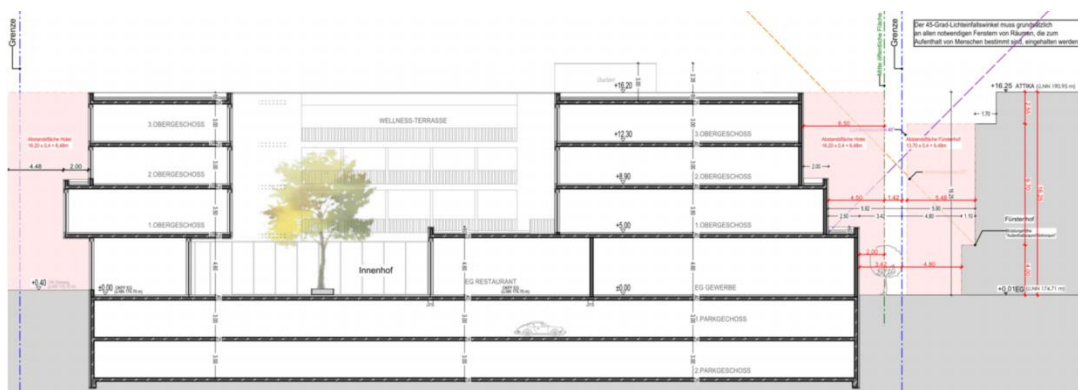
Abb. 5: Gebäudeschnitt (Stand Jan. 2021)
