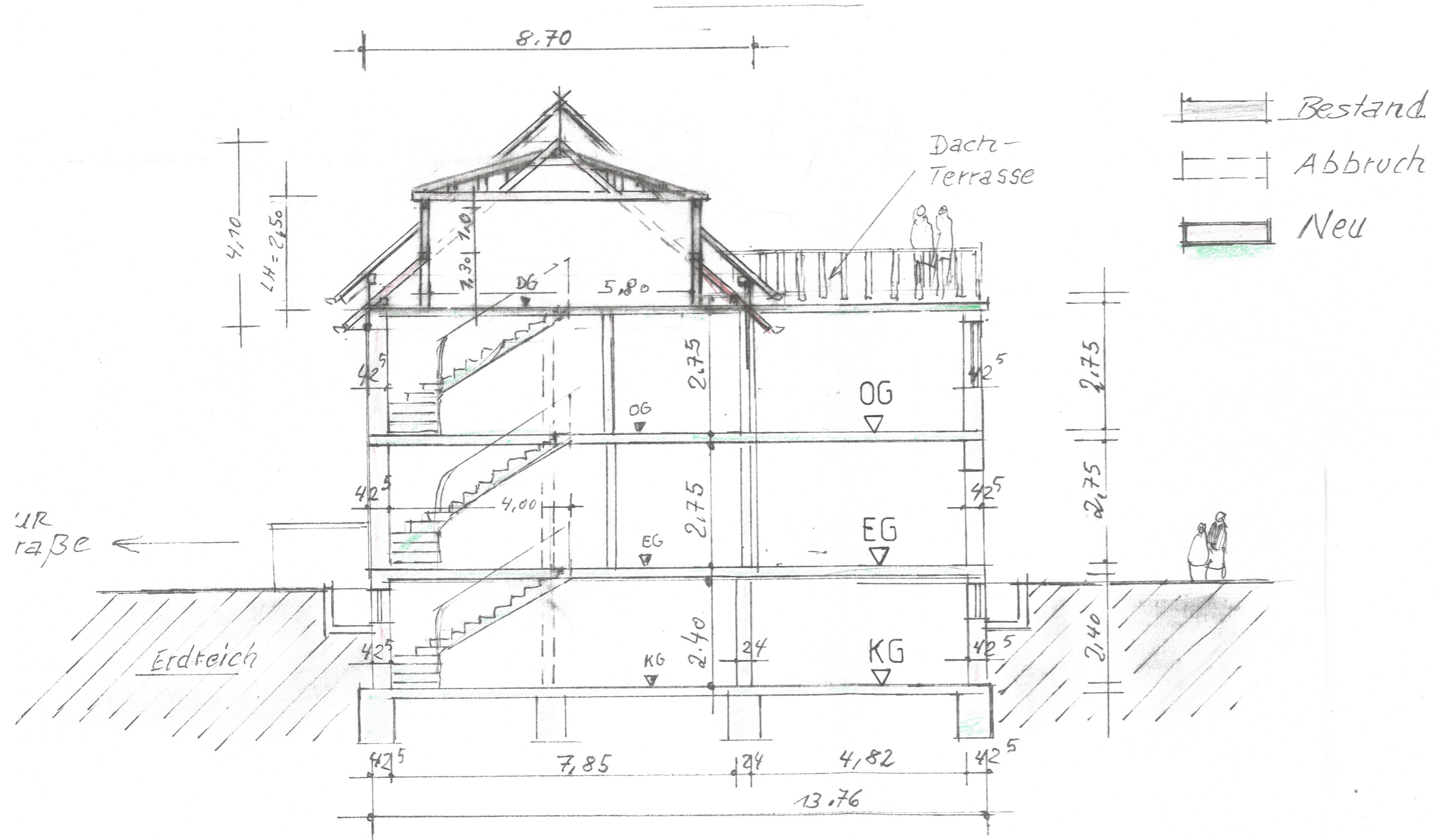
Schnitt A-B
