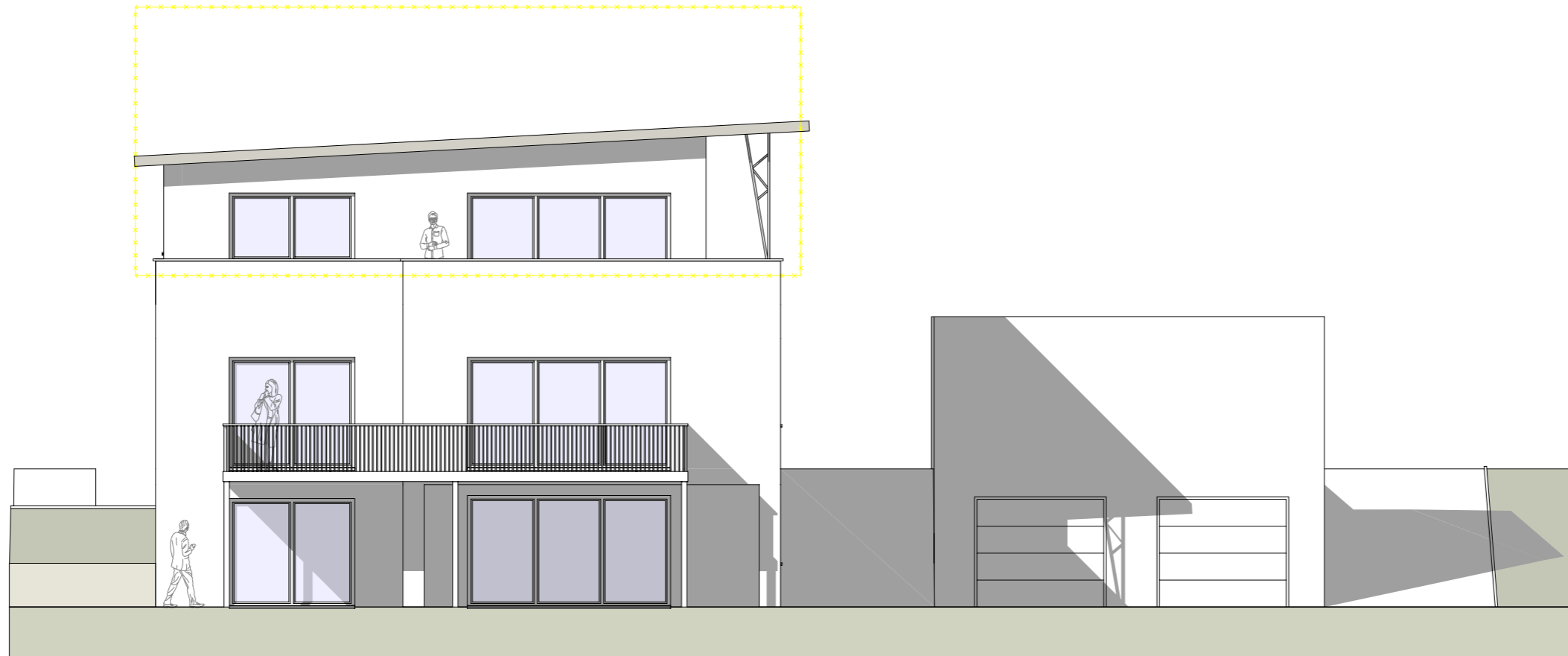
Süd-Ost-Ansicht
