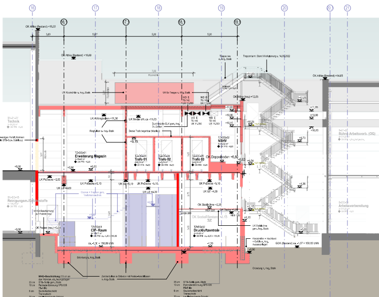
TZ_SCHN_Längs
