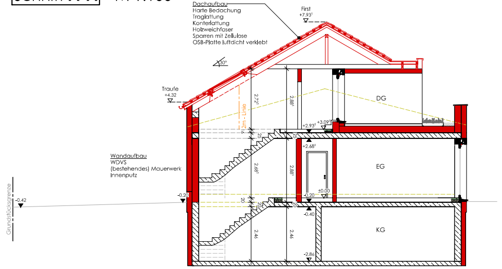
Schnitt B-B - M 1:100
