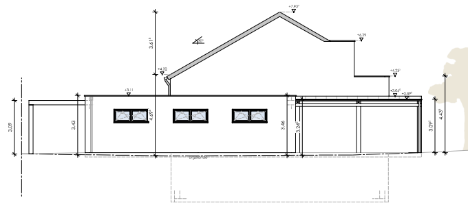
Ansicht Norden - M 1:100
