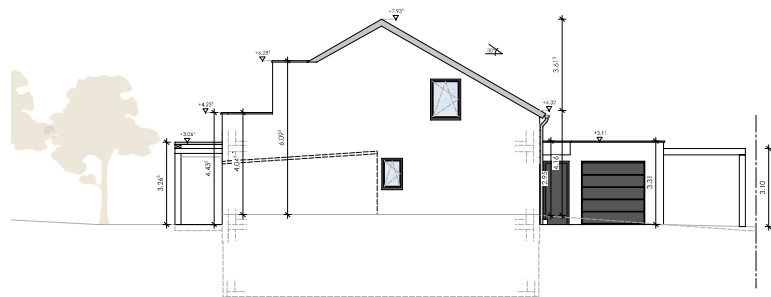
Ansicht Süden - M 1:100
