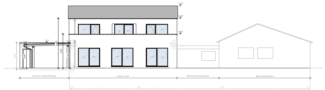
Ansicht Westen - M 1:100
