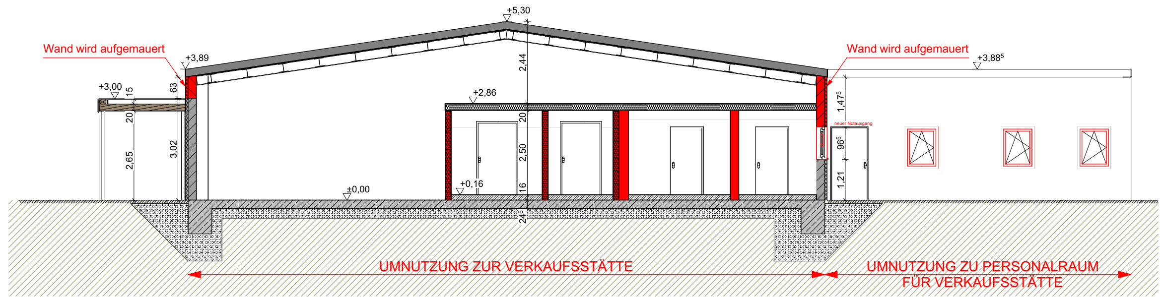
Schnitt A-A
