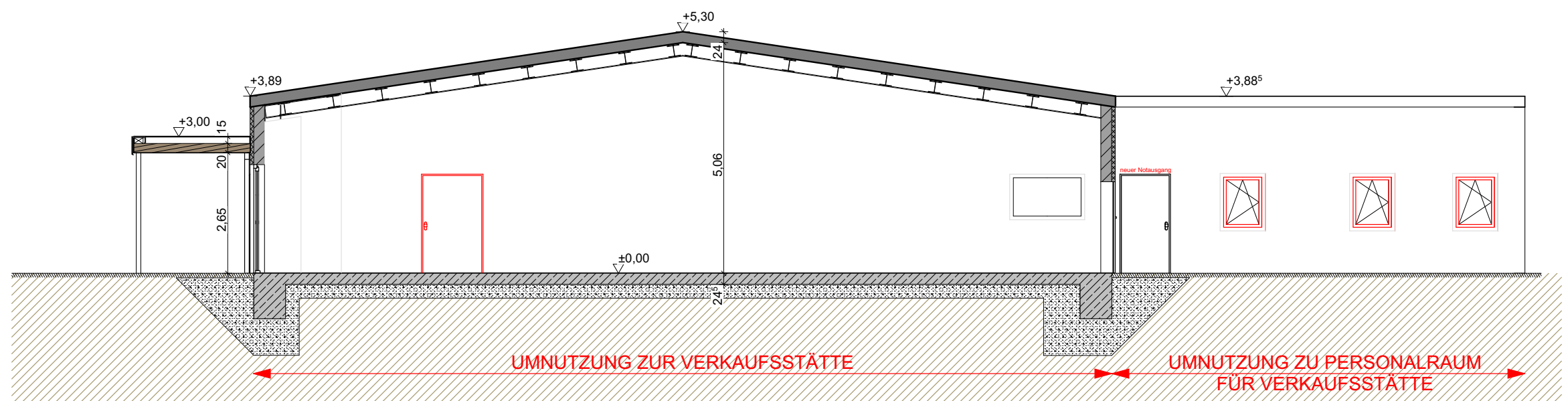
Schnitt B-B
