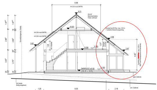
SCHNITT WOHNHAUS
