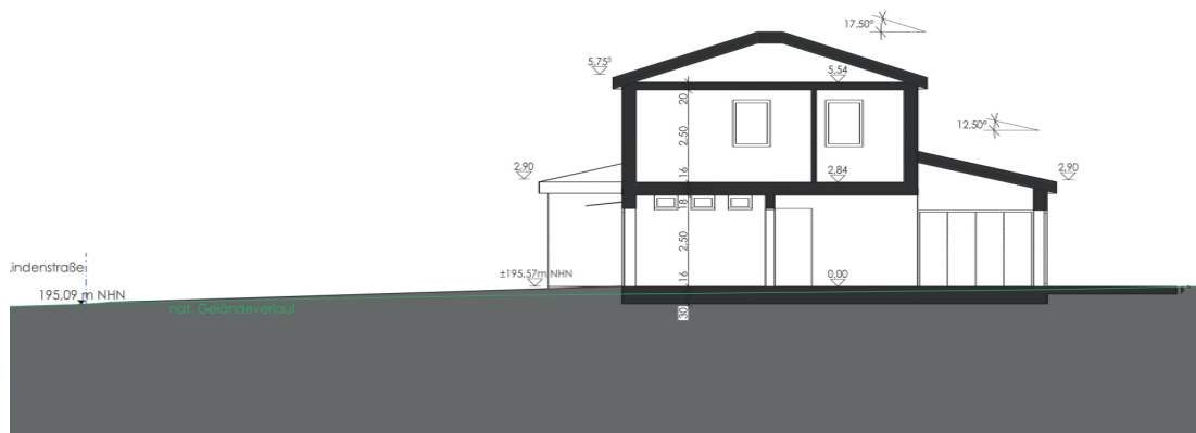
Schnitt B-B
