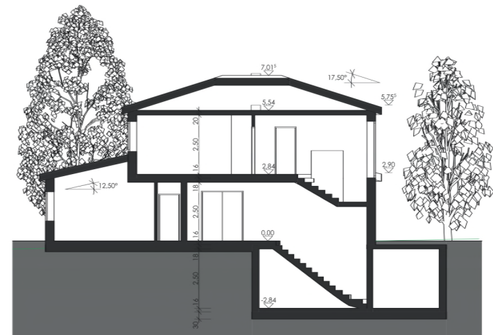
Schnitt A-A
