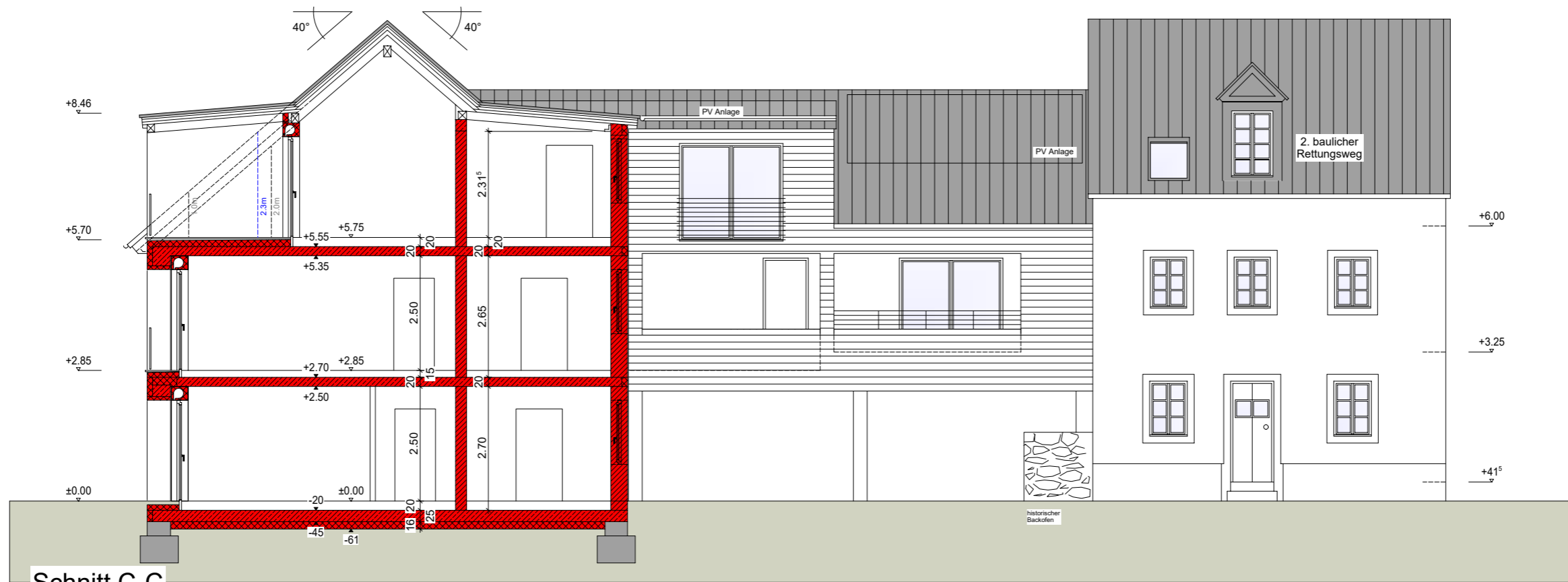
Schnitt C-C
