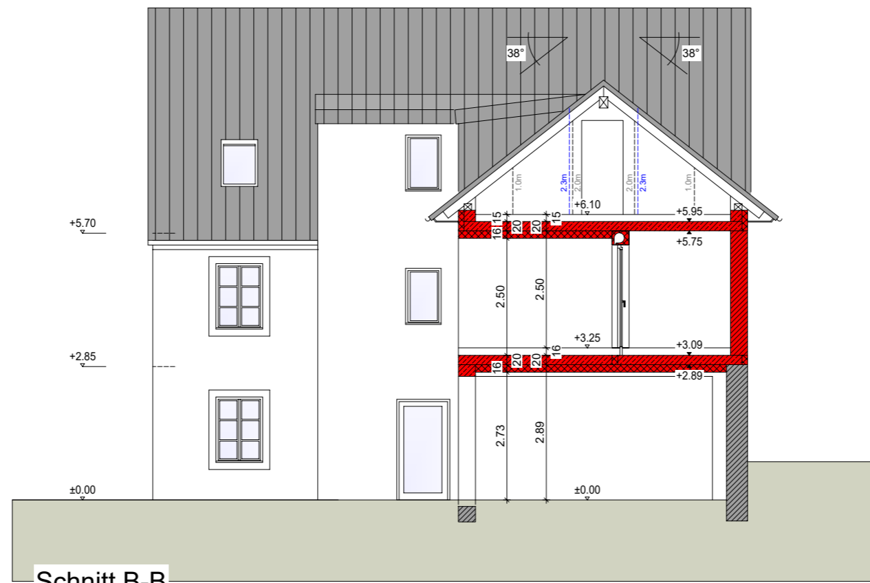
Schnitt B-B
