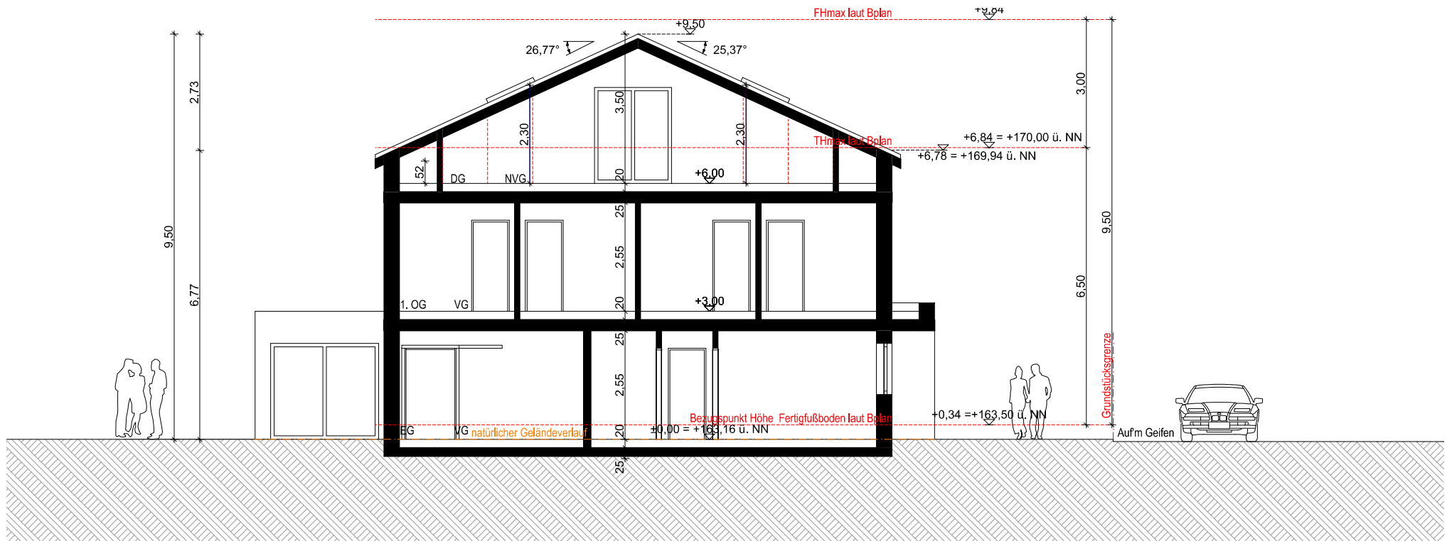
SCHNITT A-A
