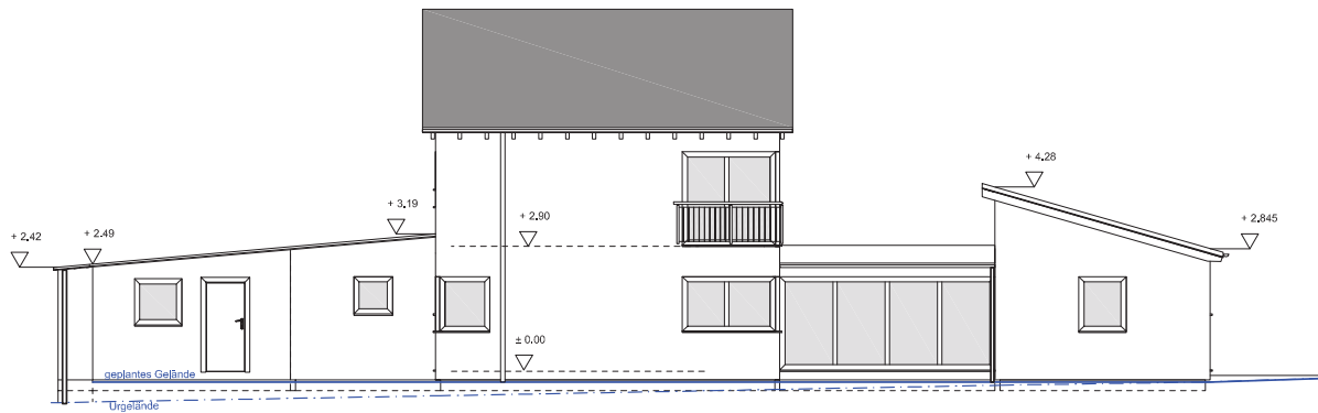
Ansicht Nord-Ost
