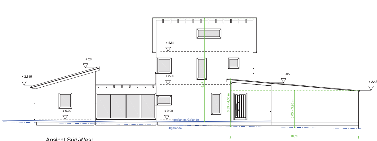
Ansicht Süd-West
