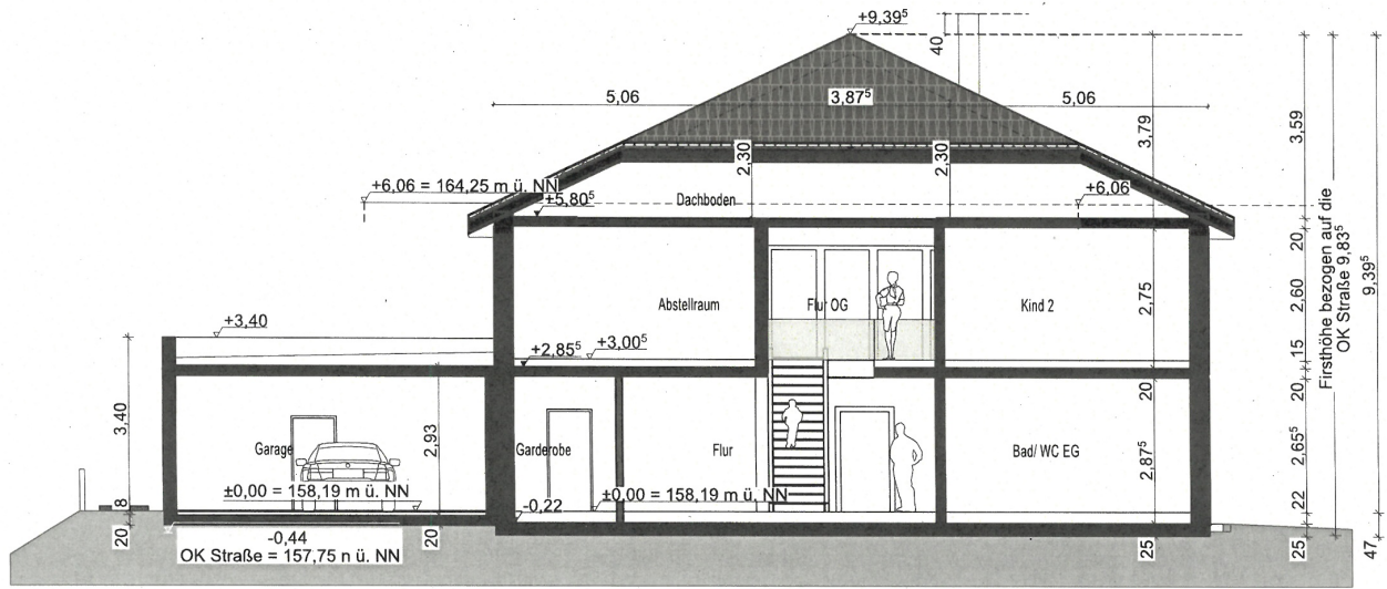
Schnitt B
