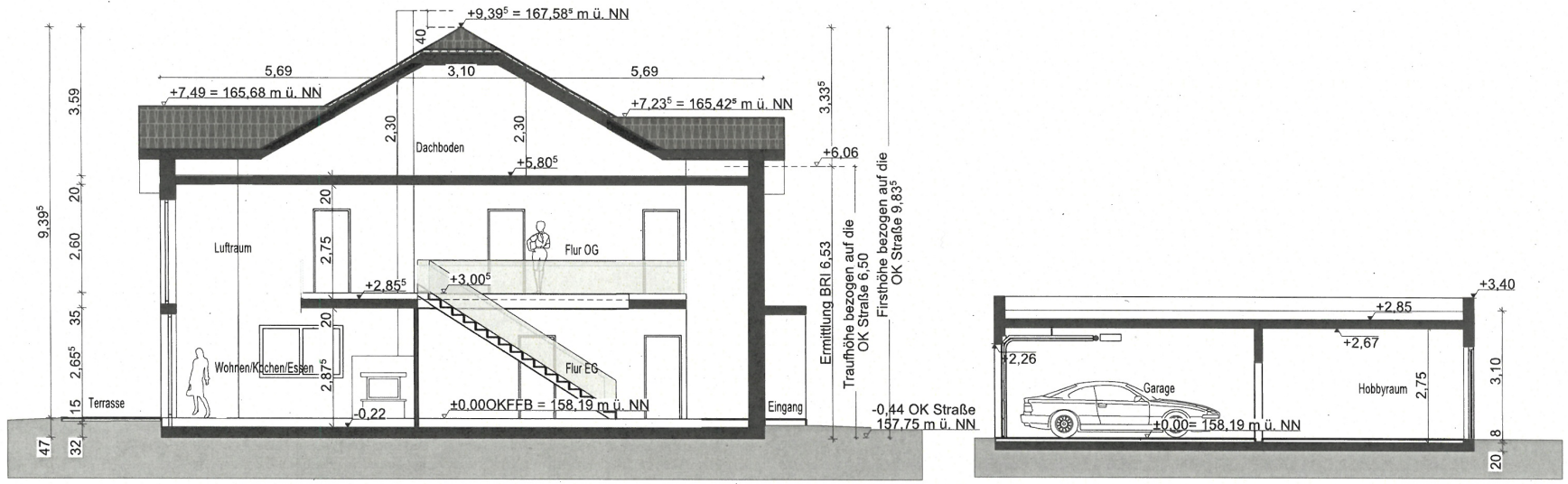
Schnitt A
