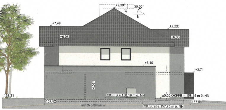
Süd-West Ansicht
