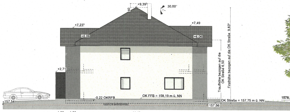
Nord-Ost Ansicht
