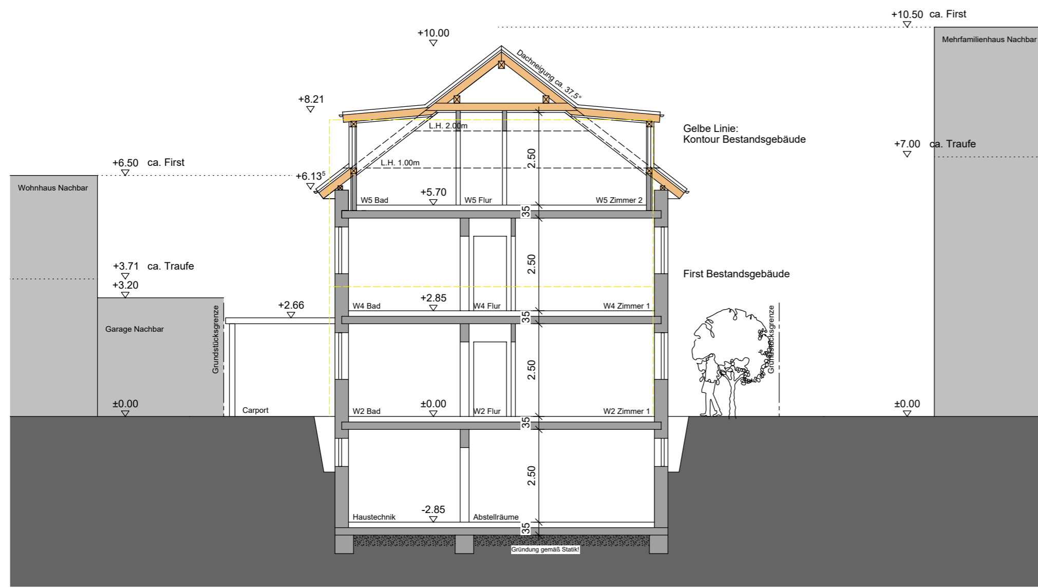
Schnitt A-A
