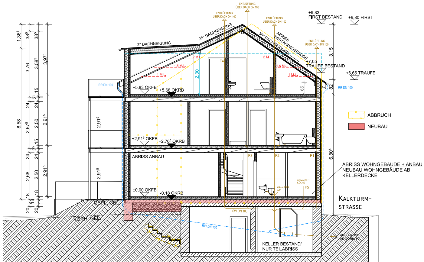
Schnitt A-A
