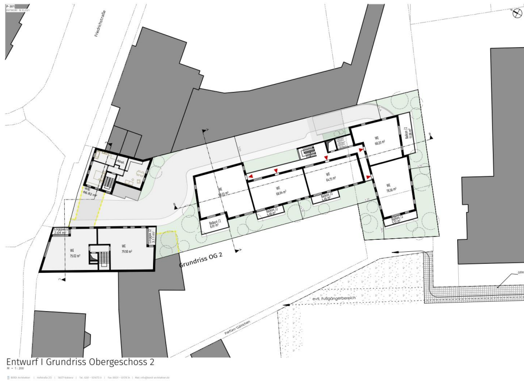
Abb. 8: 2. Obergeschoss
