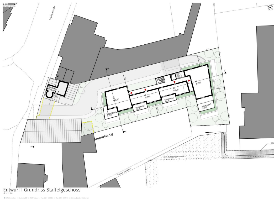
Abb. 9: Staffelgeschoss
