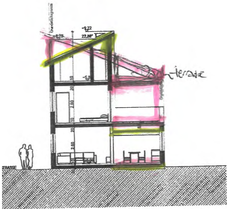
SCHNITT A-A 1.100
