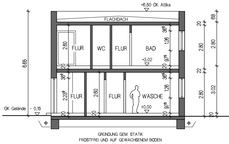
SCHNITT A-A
