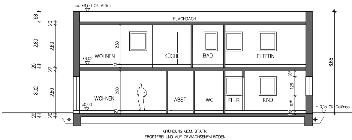
SCHNITT B-B
