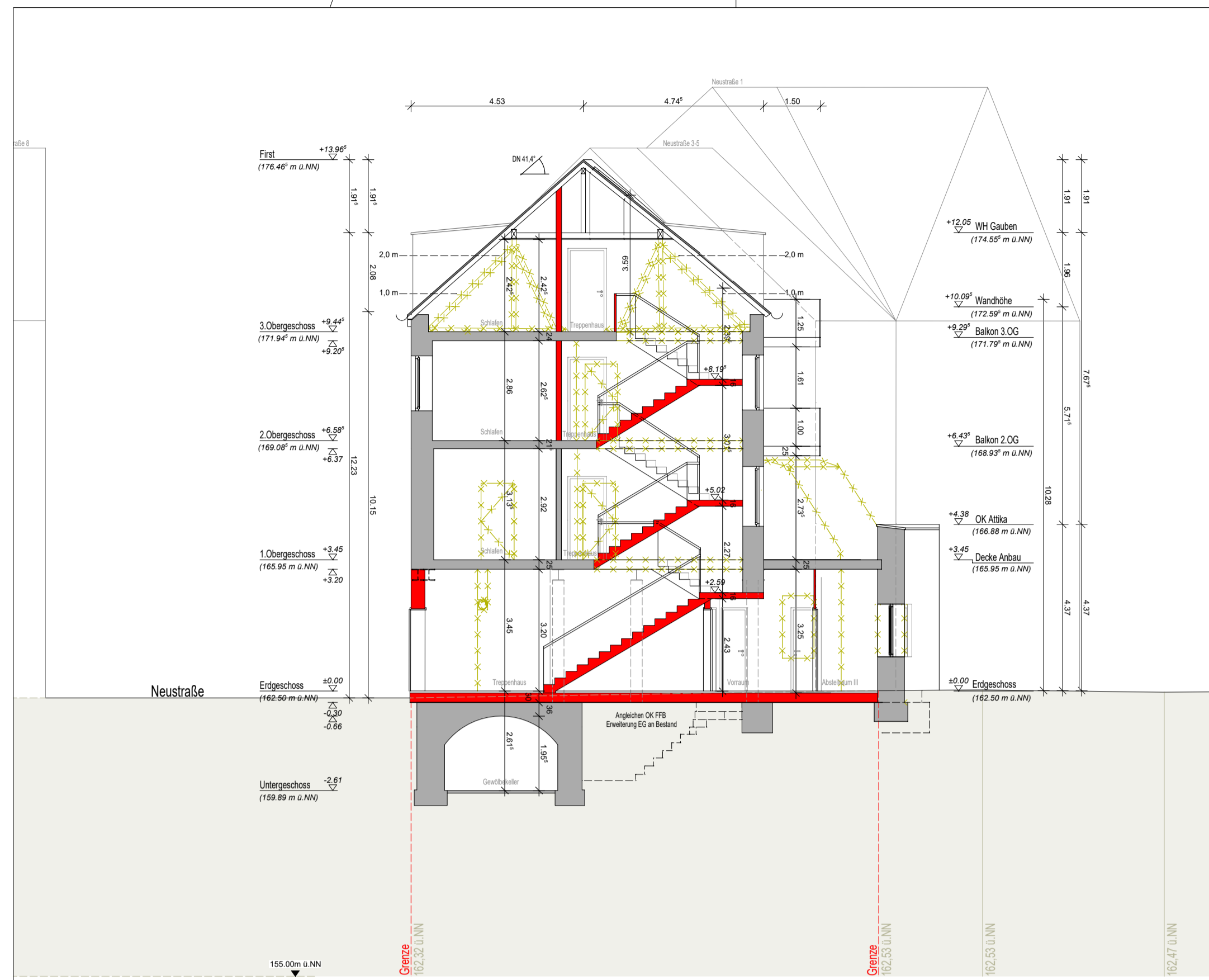
Schnitt A
