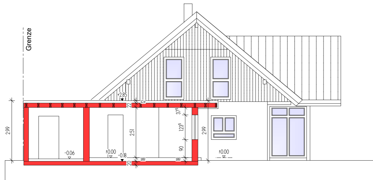
Schnitt A-A
