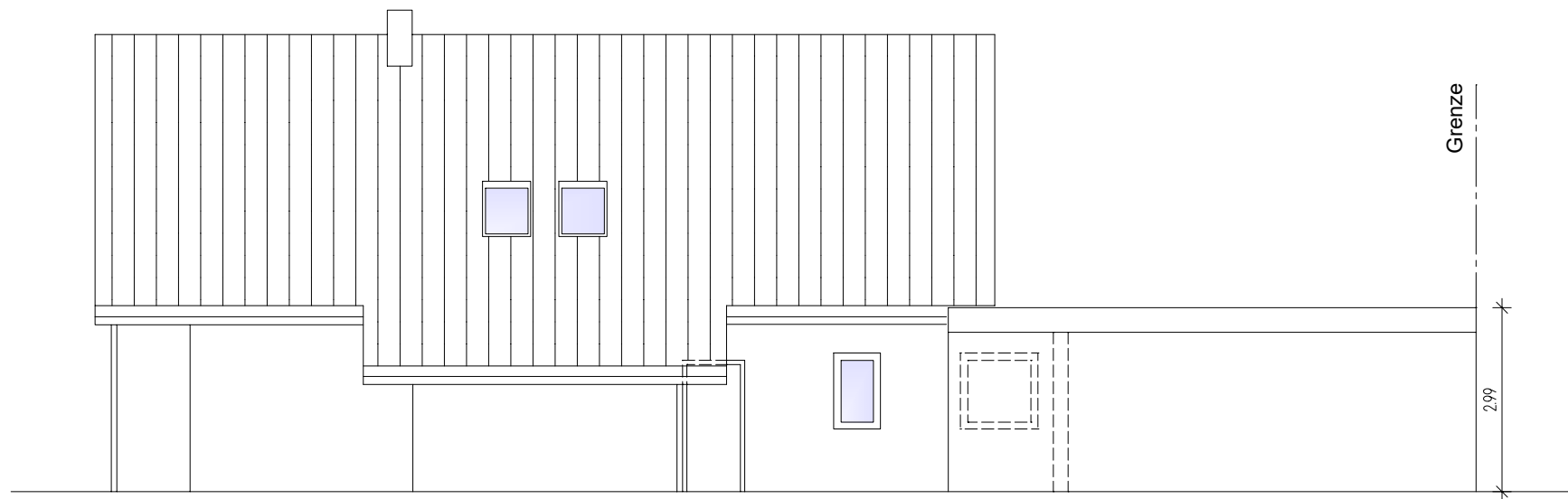
Nordansicht
