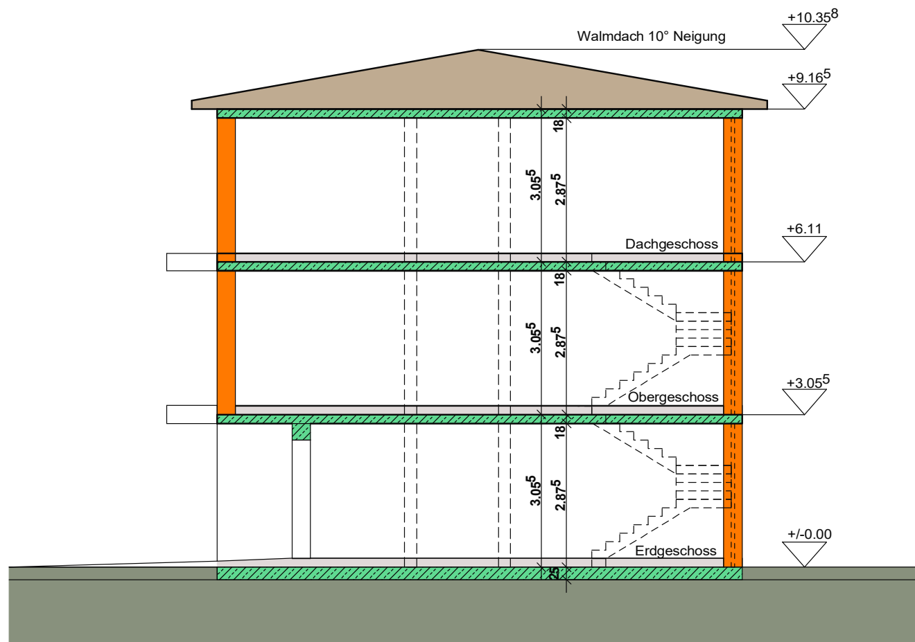
Querschnitt im M.: 1//100
