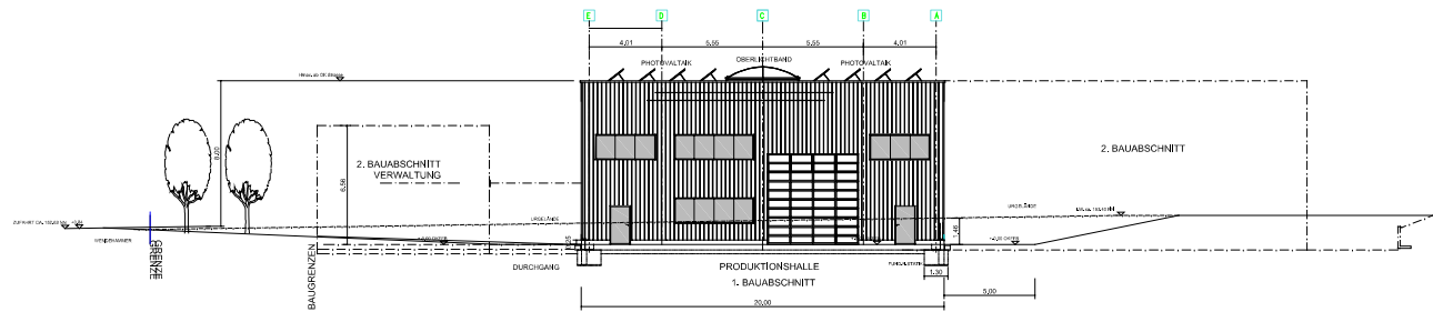
OST ANSICHT
