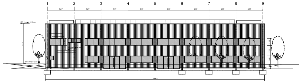
SÜD ANSICHT
