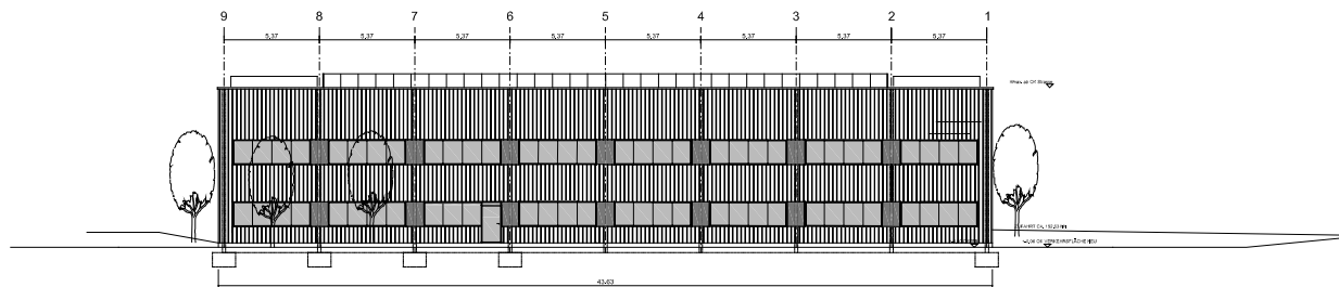
NORD ANSICHT
