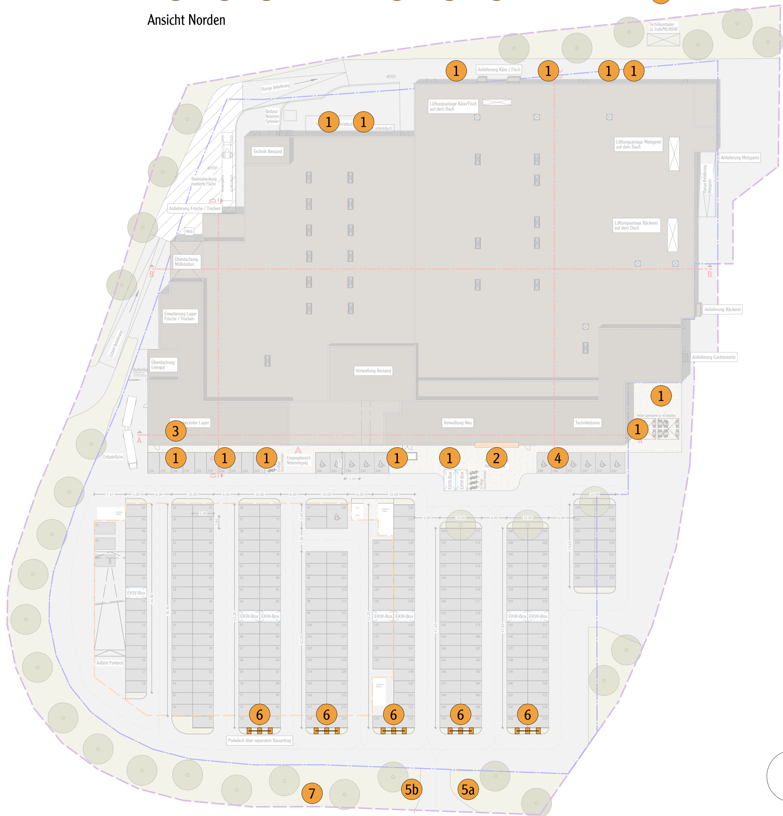
Freiflächenplan mit Positionierung der Werbeanlagen
