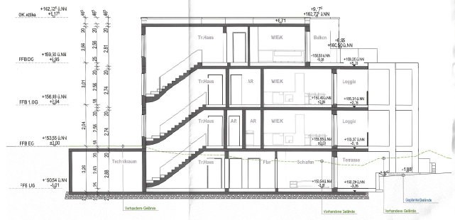
SCHNITT 2-2
