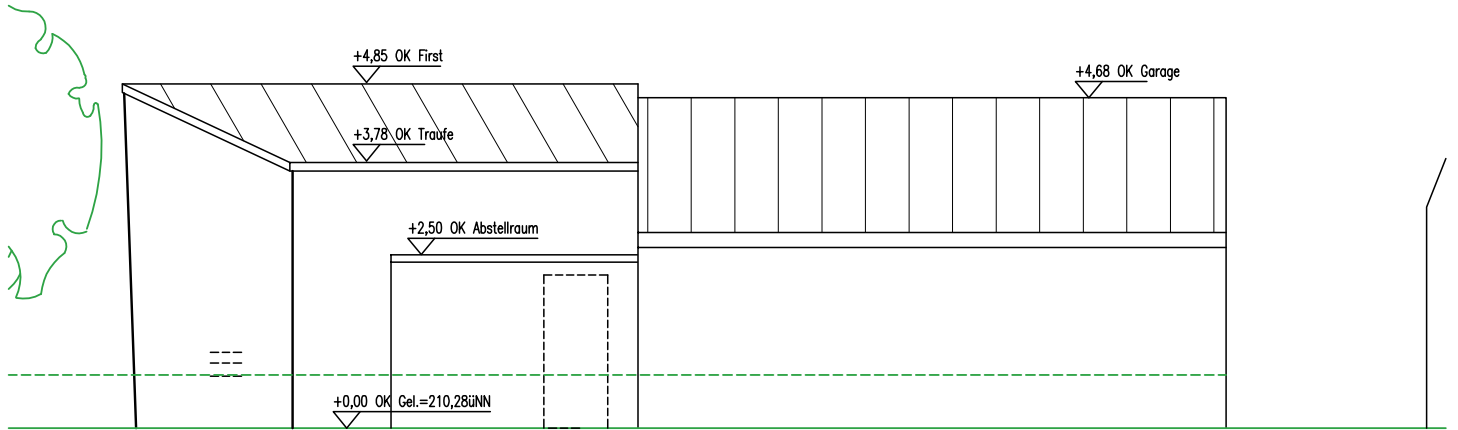
Rückansicht
