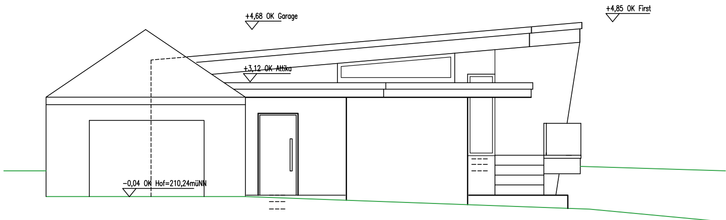
Ansicht Eingang
