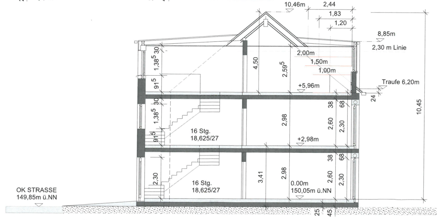
SCHNITT B-B
