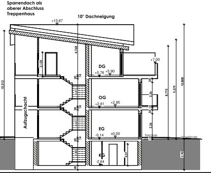
SCHNITT
