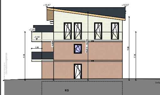
ANSICHT NORD-WEST
