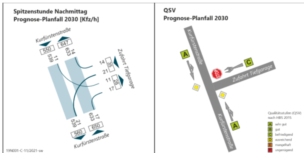
Bild 5: Knotenstromdarstellung und Verkehrsqualität in der nachmittäglichen Spitzensunde am Knotenpunkt Kurfürstenstraße / Zufahrt Tiefgarage (KP01) im Prognose-Planfall 2030
