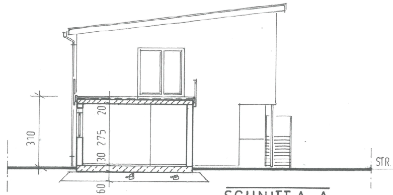
SCHNITT A-A
