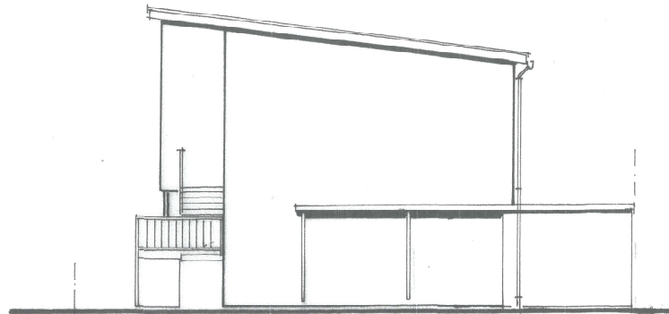
SÜDANSICHT
