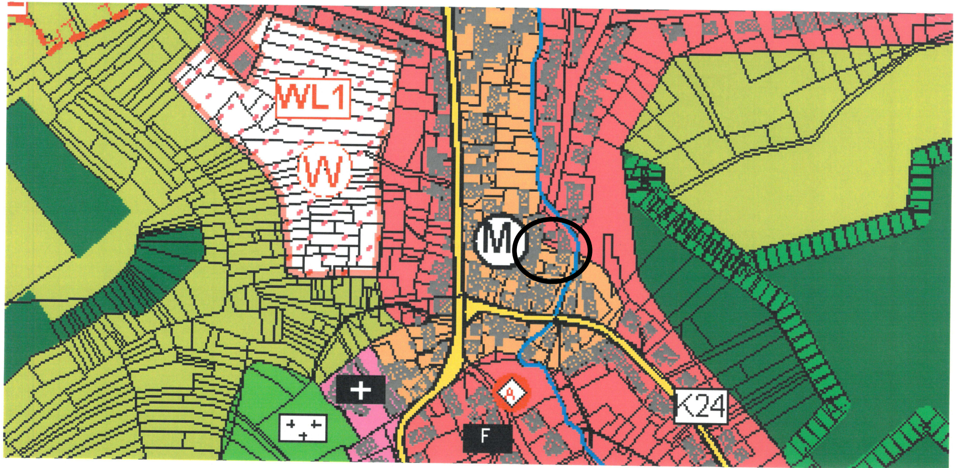
Auszug Flächennutzungsplan
