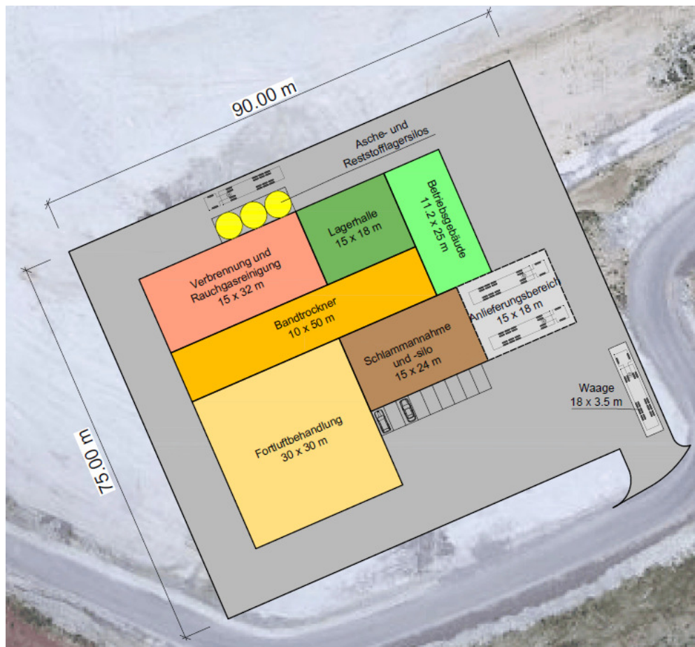
Abbildung 1: Lageplankonzept für eine zentrale Lösung
