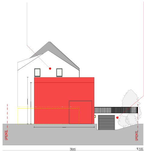
Nord 1:100
