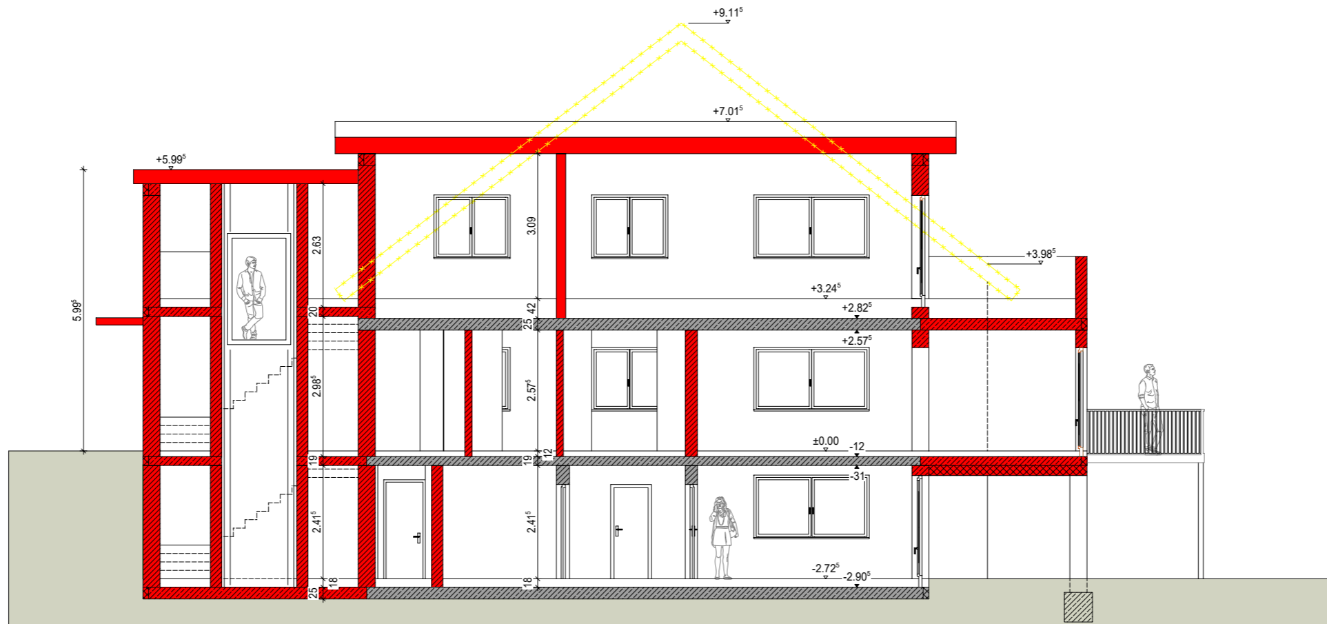
Schnitt
