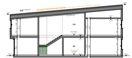
SCHNITT A-A (Bürogebäude)
