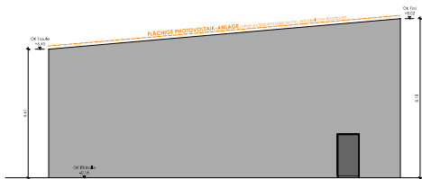
ANSICHT SÜD-OST
