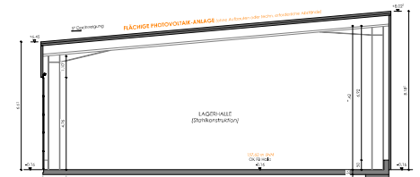
SCHNITT B-B (Lagerhalle)
