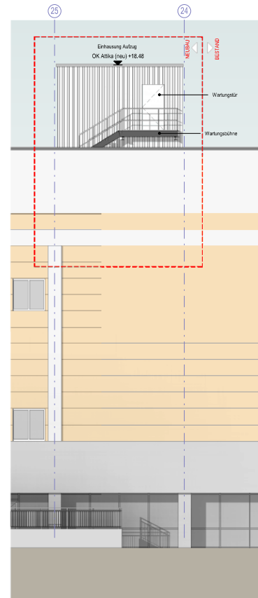
Ansicht Nord_Einhausung (Aufzug)
