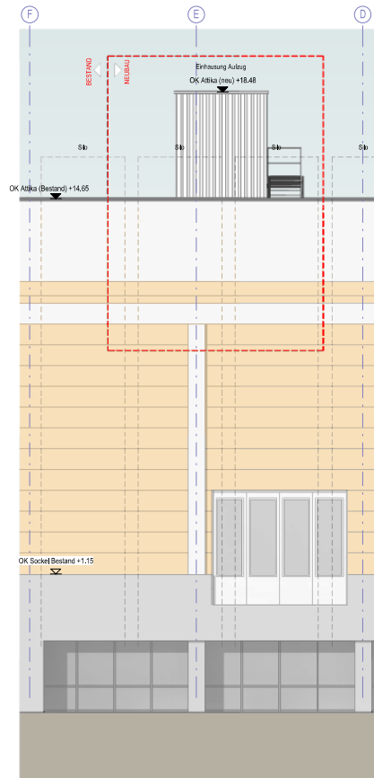
Ansicht Ost_Einhausung (Aufzug)
