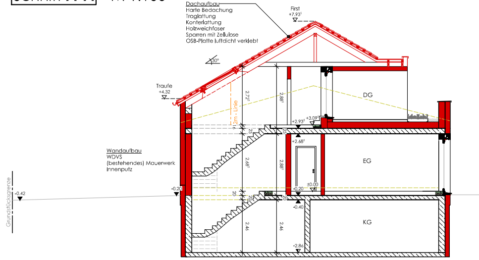
Schnitt B-B - M 1:100
