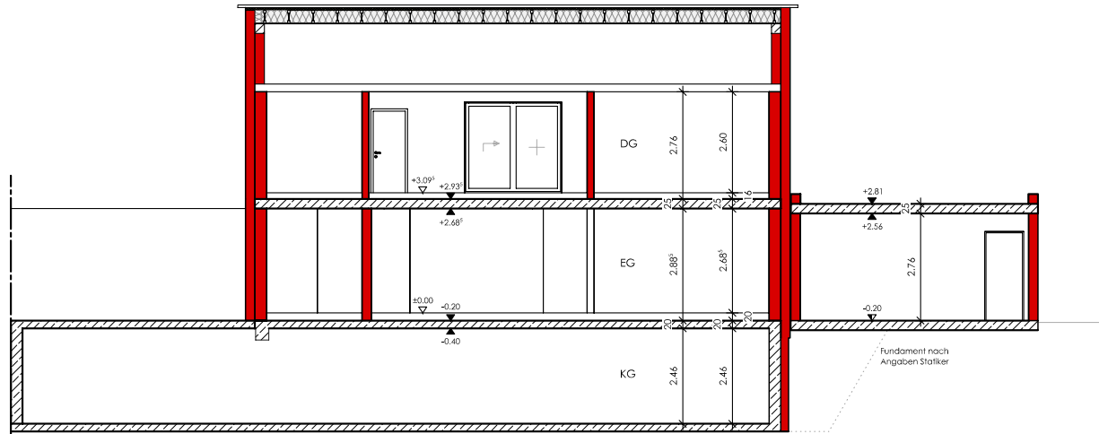
Schnitt A-A - M 1:100
