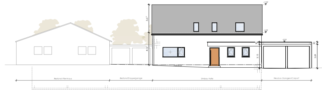
Ansicht Osten - M 1:100
