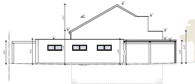
Ansicht Norden - M 1:100
