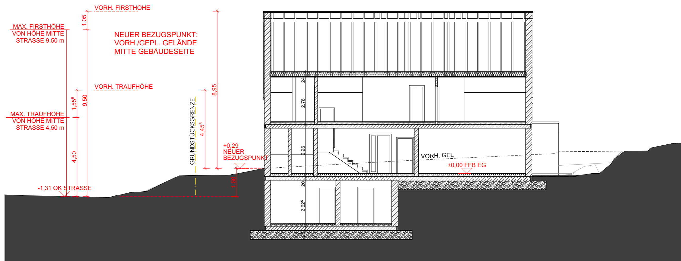
Schnitt B-B
