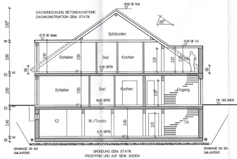
SCHNITT B-B
