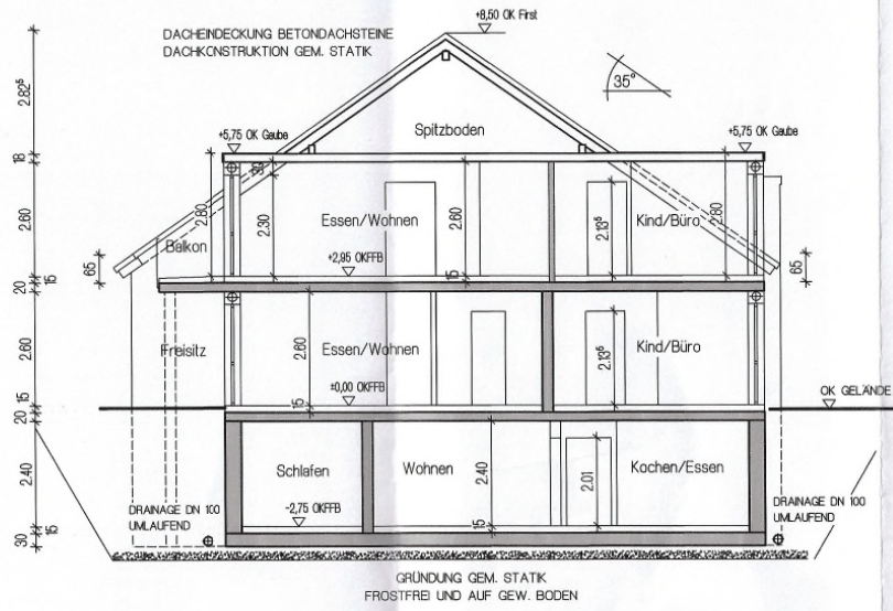
SCHNITT A-A
