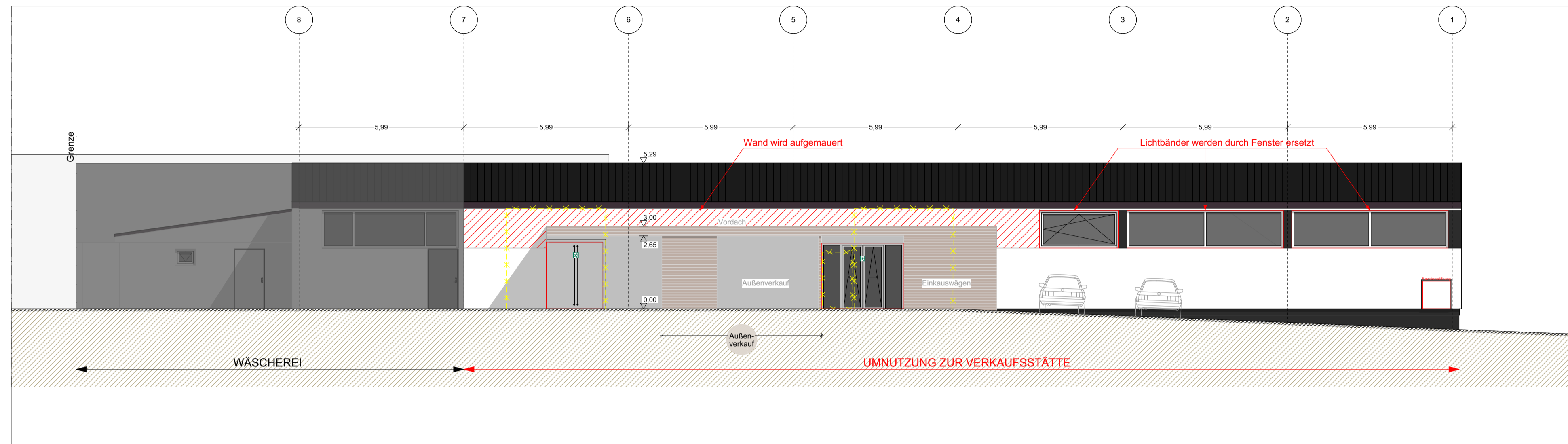
ANSICHT WEST
