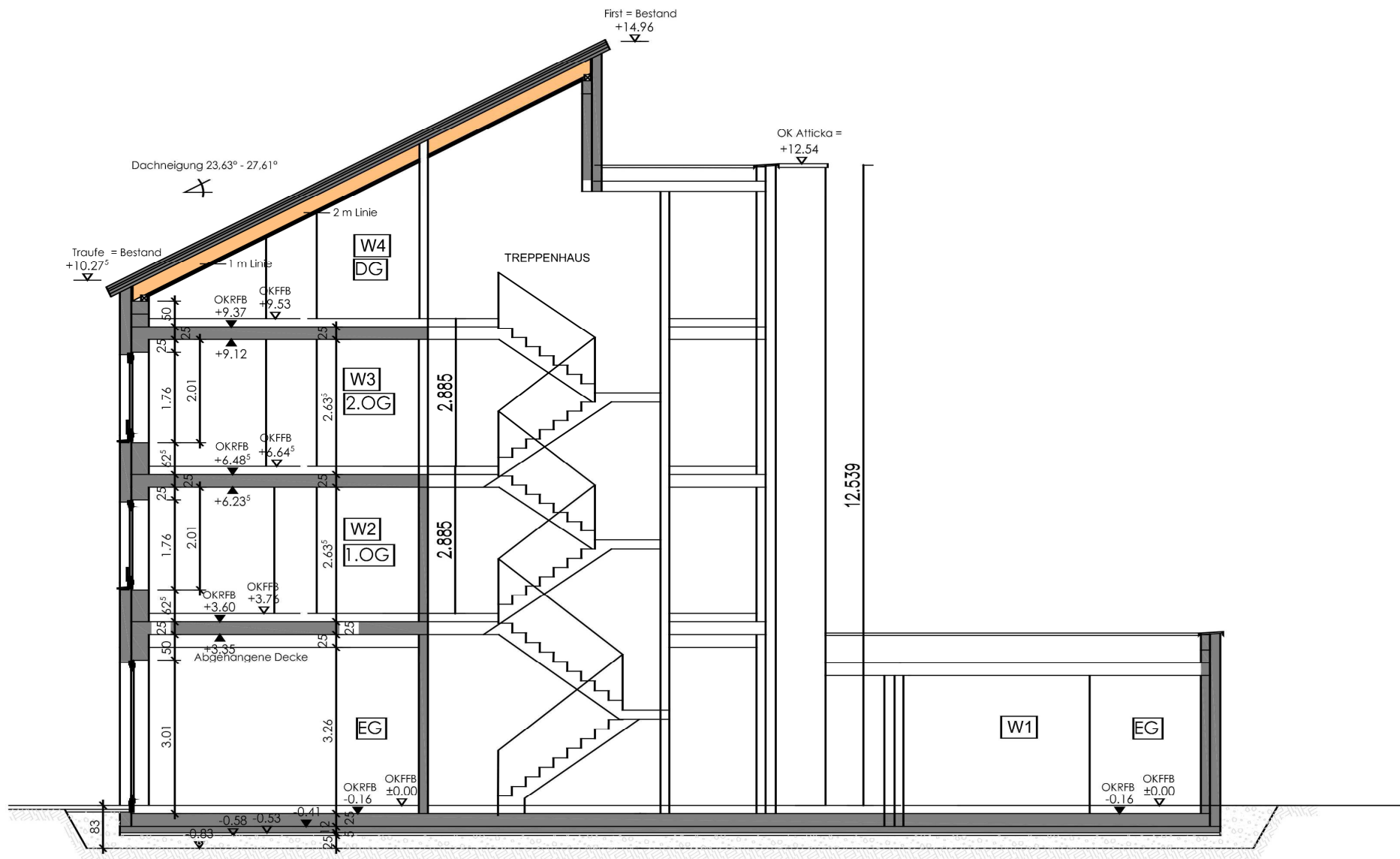
SCHNITT A-A
