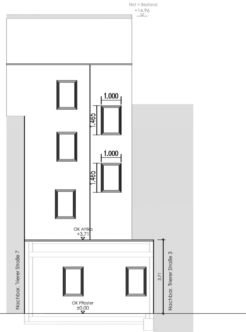
RÜCKSEITE
