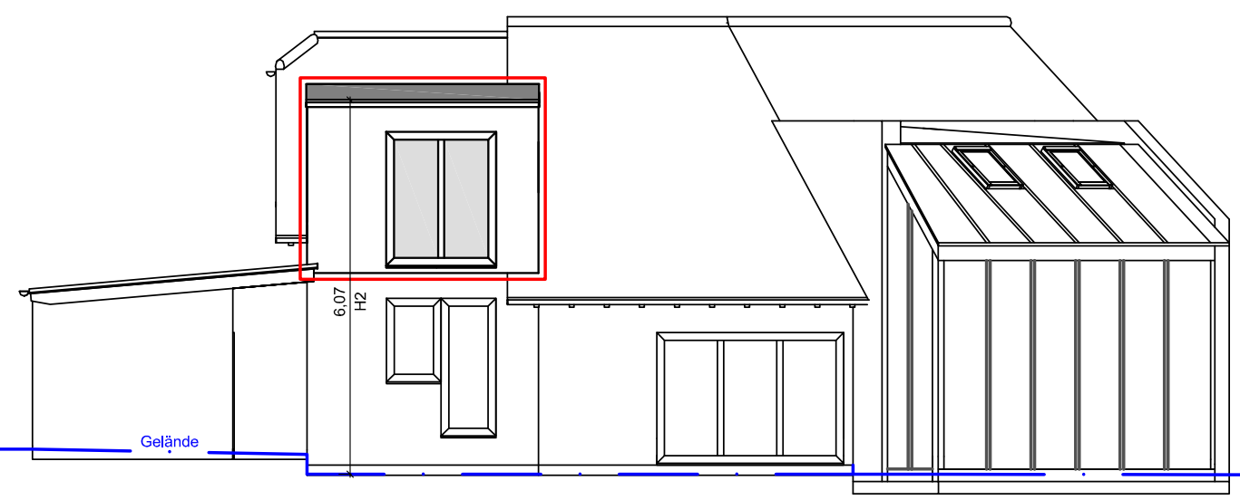
Ansicht Süd
