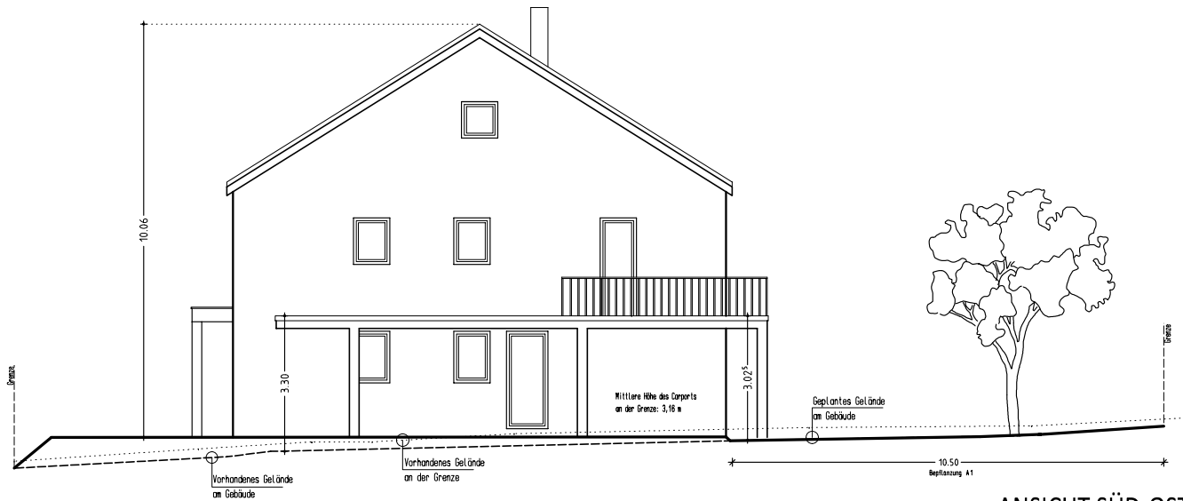
ANSICHT SÜD-OST
