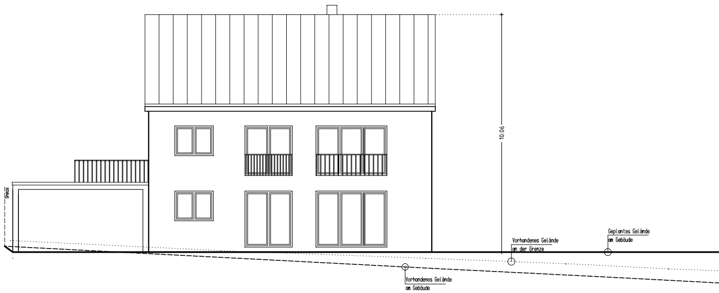
ANSICHT NORD-OST
