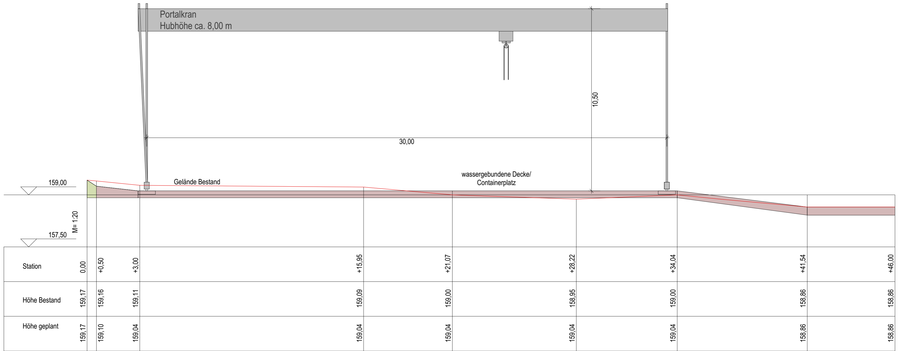
M= 1:100 Schnitt A-A
