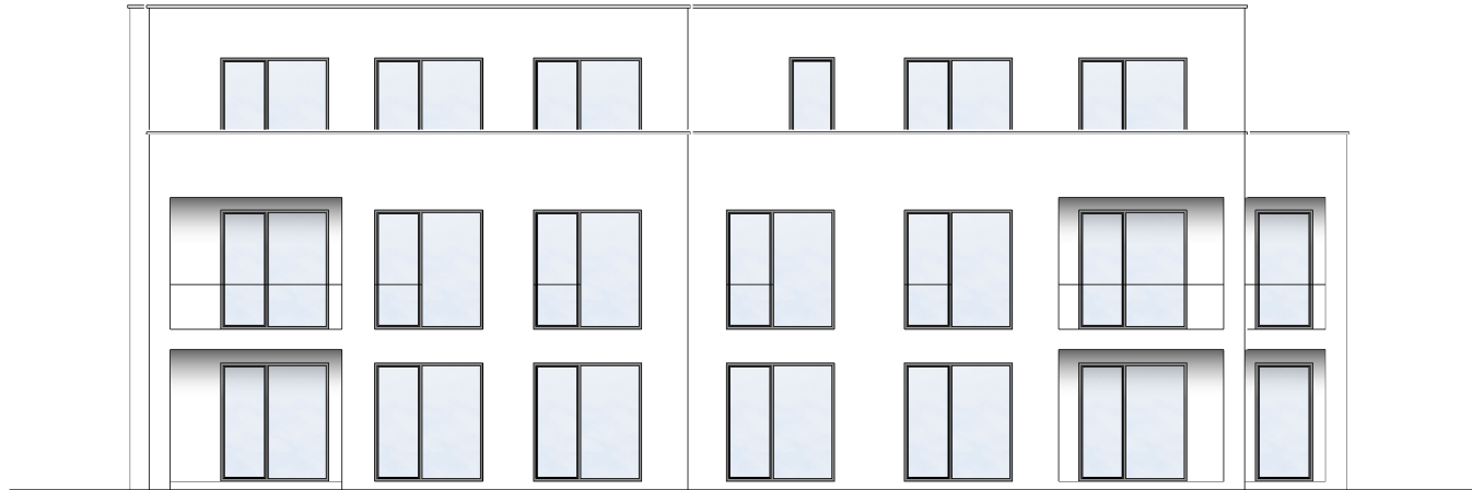
Ansicht Süd-West
