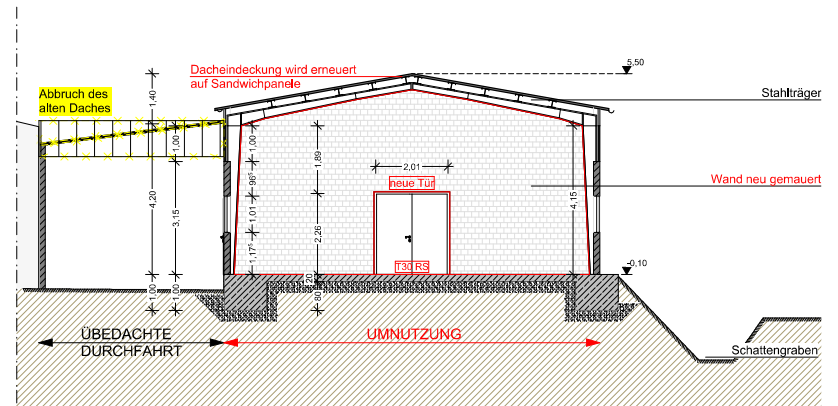
SCHNITT A-A
