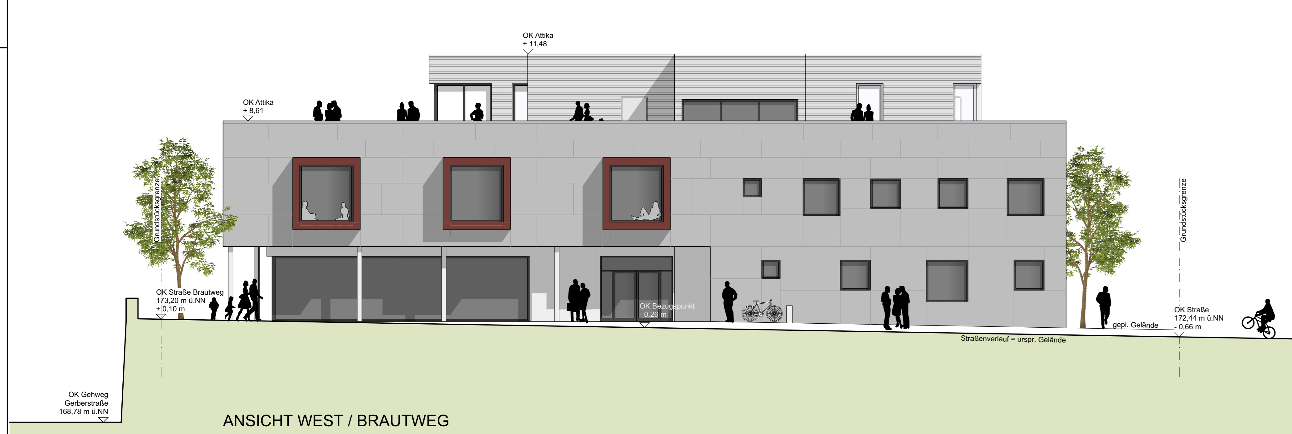
ANSICHT WEST / BRAUTWEG
