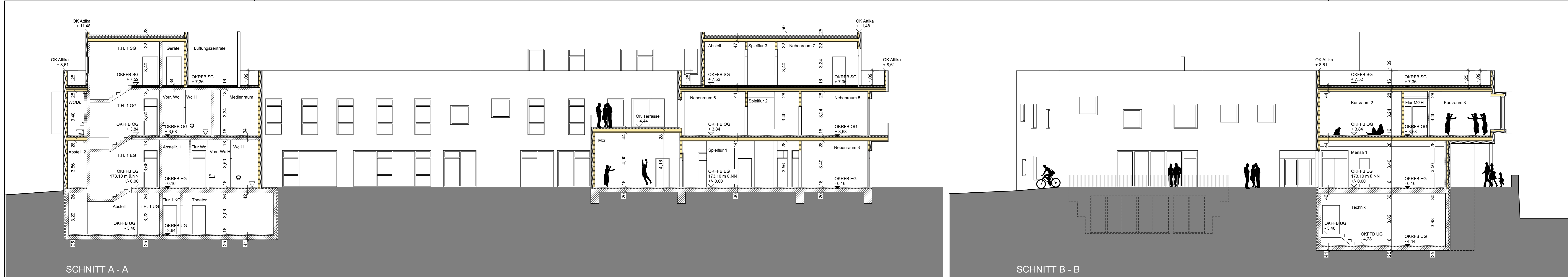
SCHNITT A - A
